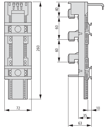
PKZM0-XC45L
