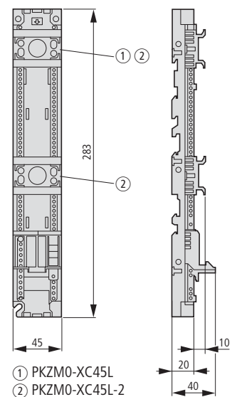
PKZM0-XC45L-2
